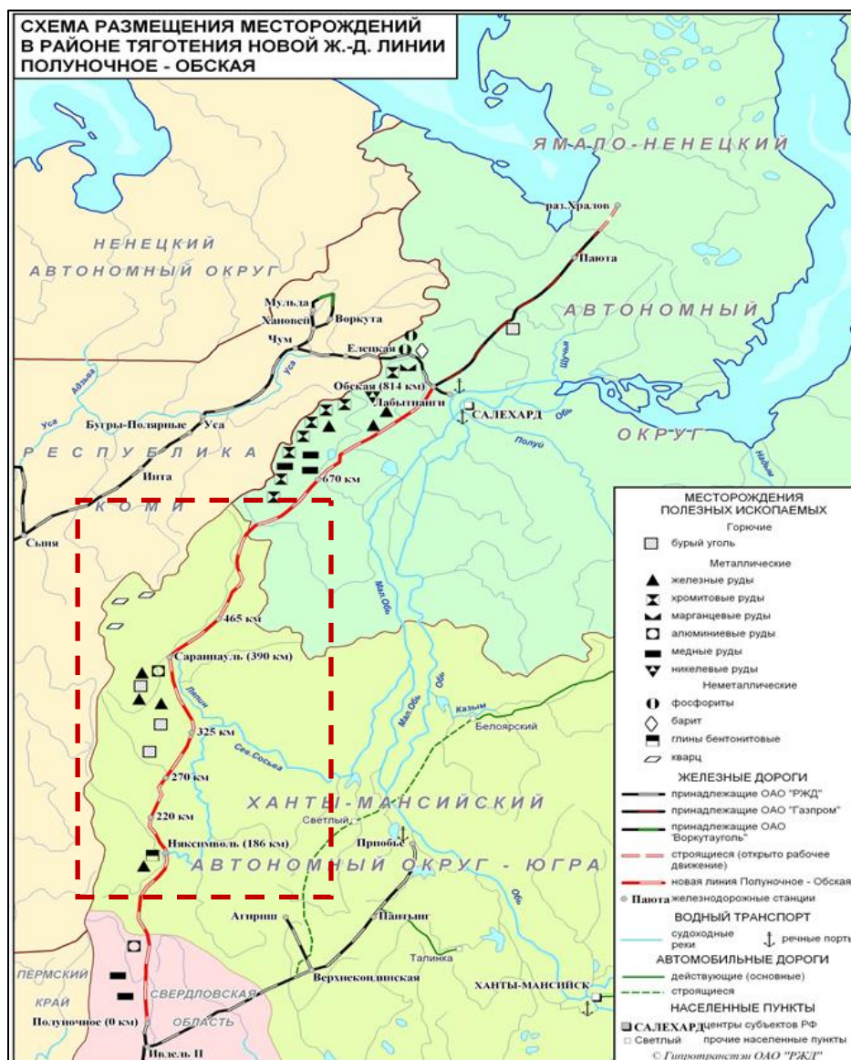
Рисунок 4.3.1 – Схема ж/д линии Полуночное – Обская
